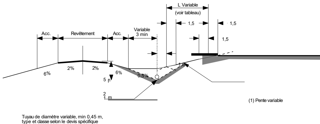
PROFIL EN LONG EN DÉBLAI
