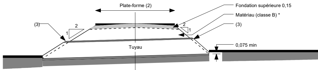
Figure 16.10.1 : Profil
